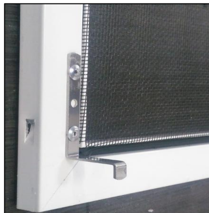
Afbeelding 2 korte montage haak aan de onderzijde
